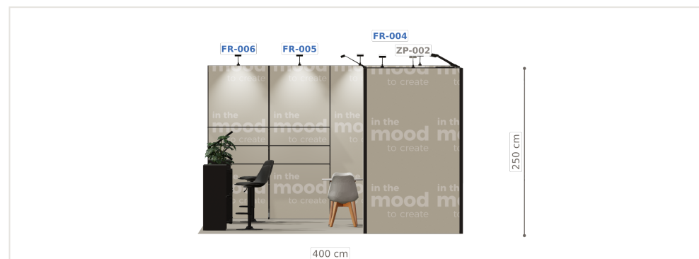
ELEWACJA 2
