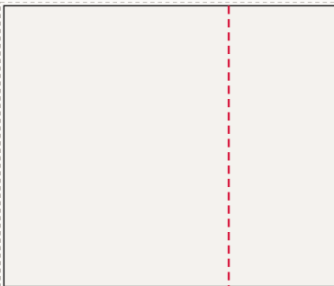
Ściana lewa od lewej: FR-005, FR-004 295 × 250 cm plik 298 × 253 cm, spad 1,5 cm po obrysie, łączeń: 1
