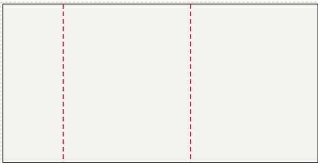
Ściana tylna od lewej: FR-001 ... FR-003 496 × 250 cm plik 499 × 253 cm, spad 1,5 cm po obrysie, łączień: 2
