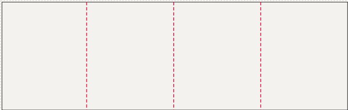
Ściana tylna od lewej: FR-001 ... FR-004 796 × 250 cm plik 799 × 253 cm, spad 1,5 cm po obrysie, łączący: 3
