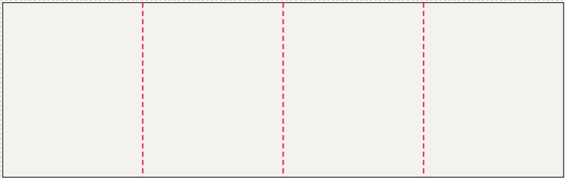
Ściana tylna od lewej: FR-001 ... FR-004 801 × 250 cm plik 804 × 253 cm, spad 1,5 cm po obrysie, łączień: 3
