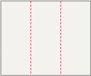
Regal Faro, strona A od lewej: IN-001 ... IN-003 300 × 250 cm plik 303 × 253 cm, spad 1,5 cm po obrysie, łączni: 2
