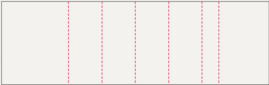
Ściana tylna od lewej: FR-002 ... FR-008 800 × 250 cm plik 803 × 253 cm, spad 1,5 cm po obrysie, łączęci: 6
