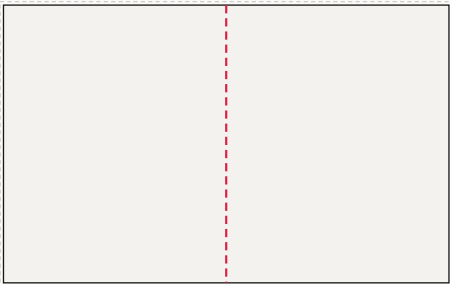
Ściana lewa od lewej: FR-011, FR-010 401 × 250 cm plik 404 × 253 cm, spad 1,5 cm po obrysie, łączęci: 1
