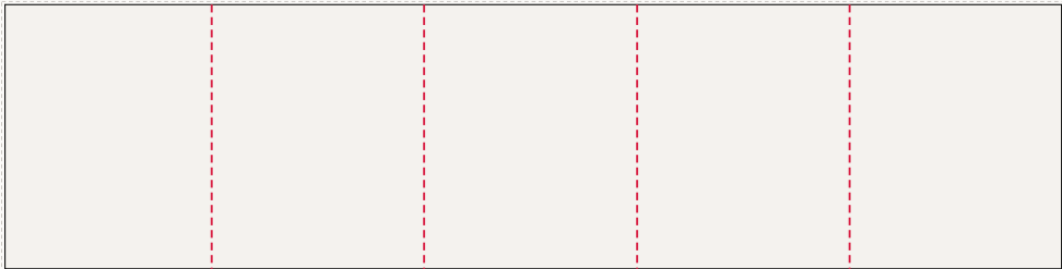
Ściana tylna od lewej: FR-001 ... FR-005 997 × 250 cm plik 1000 × 253 cm, spad 1,5 cm po obrysie, łączeń: 4
