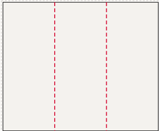
Regał Faro, strona A od lewej: IN-001 ... IN-003 300 × 250 cm plik 303 × 253 cm, spad 1,5 cm po obrysie, łączę: 2
