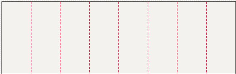
Ściana tylna od lewej: FR-001 ..., FR-008 800 × 250 cm plik 803 × 253 cm, spad 1,5 cm po obrysie, łączeń: 7
