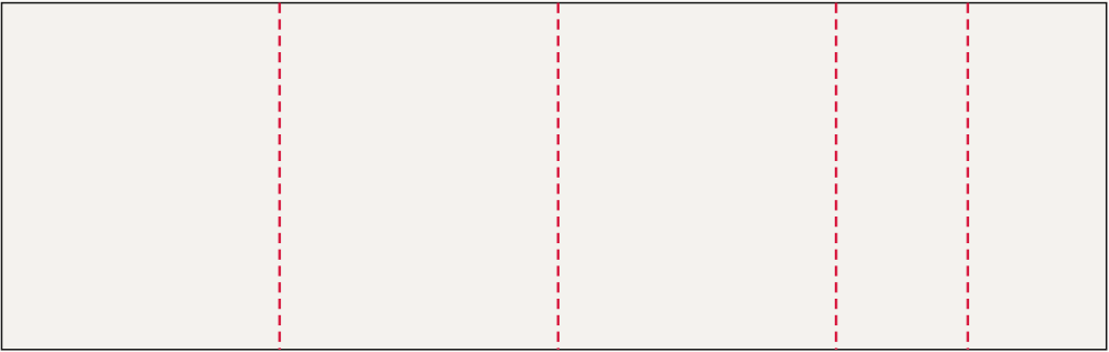
Ściana tylna od lewej: FR-002 ... FR-006 797 × 250 cm plik 800 × 253 cm, spad 1,5 cm po obrysie, łączęń: 4
