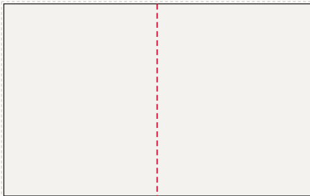
Ściana tylna, część 2 z 2 od lewej: FR-004, FR-005 400 × 250 cm plik 403 × 253 cm, spad 1,5 cm po obrysie, łączeń: 1
