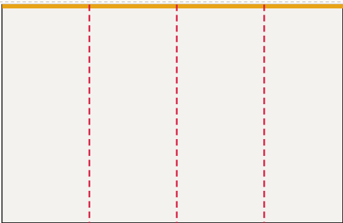
Ściana lewa od lewej: FR-009 ... FR-006, LED 390 × 250 cm plik 393 × 253 cm, spad 1,5 cm po obrysie, łączeń: 3
