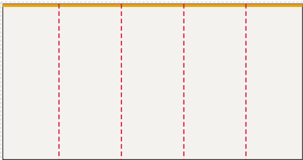
Ściana tylna od lewej: FR-001 ... FR-005, LED 480 × 250 cm plik 483 × 253 cm, spad 1,5 cm po obrysie, łączęć: 4
