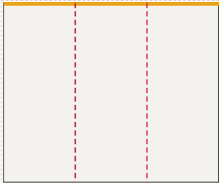
Ściana prawa od lewej: FR-006 ... FR-008, LED 300 × 250 cm plik 303 × 253 cm, spad 1,5 cm po obrysie, łączęć: 2
