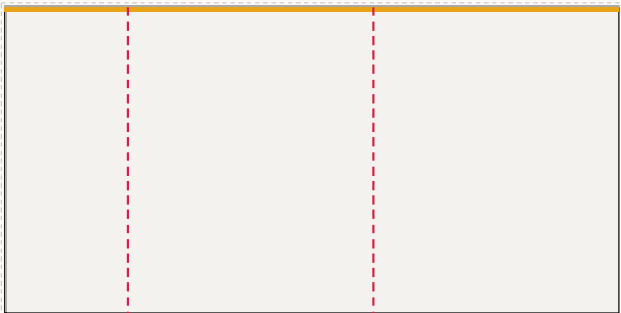
Ściana prawa od lewej: FR-004 ... FR-006, LED 500 × 250 cm plik 503 × 253 cm, spad 1,5 cm po obrysie, łączeń: 2
