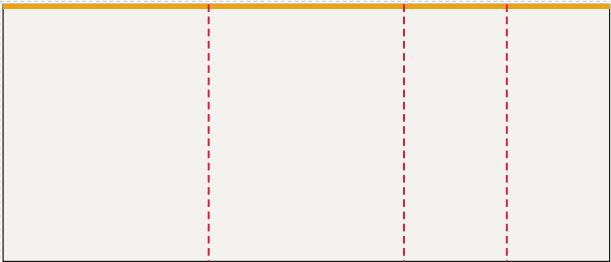
Ściana prawa od lewej: FR-005 ... FR-008, LED 590 × 250 cm plik 593 × 253 cm, spad 1,5 cm po obrysie, łączeń: 3
