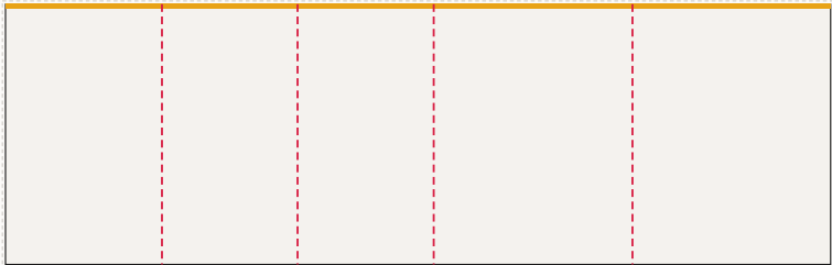
Ściana tylna od lewej: FR-001 ... FR-005, LED 791 × 250 cm plik 794 × 253 cm, spad 1,5 cm po obrysie, łączy: 4
