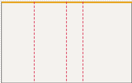
Ściana prawa od lewej: FR-004 ... FR-007, LED 400 × 250 cm plik 403 × 253 cm, spad 1,5 cm po obrysie, łączeń: 3
