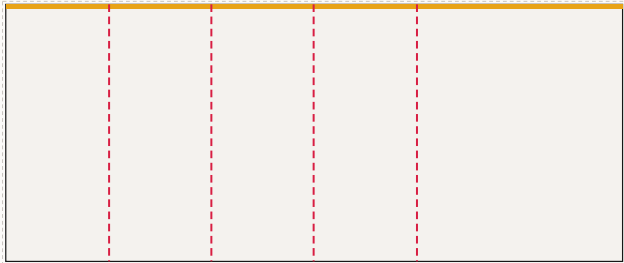
Ściana tylna od lewej: FR-001 ... FR-005, LED 600 × 250 cm plik 603 × 253 cm, spad 1,5 cm po obrysie, łączni: 4
