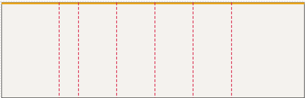
Ściana tylna od lewej: FR-001 ... FR-007, LED 790 × 250 cm plik 793 × 253 cm, spad 1,5 cm po obrysie, łączzeń: 6
