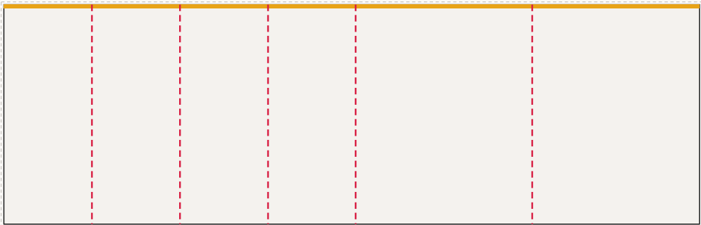
Ściana tylna od lewej: FR-001 ... FR-006, LED 790 × 250 cm plik 793 × 253 cm, spad 1,5 cm po obrysie, łączęci: 5
