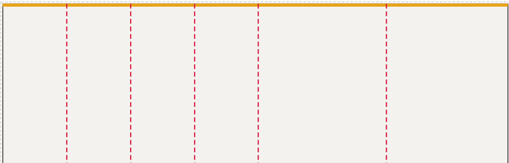
Ściana tylna od lewej: FR-001 ... FR-006, LED 790 × 250 cm plik 793 × 253 cm, spąd 1,5 cm po obrysie, łączeń: 5
