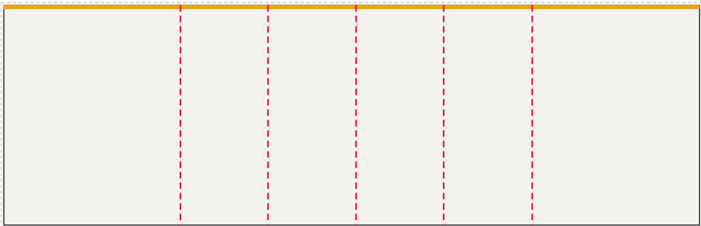
Ściana tylna od lewej: FR-001 ... FR-006, LED 790 × 250 cm plik 793 × 253 cm, spad 1,5 cm po obrysie, łączeń: 5
