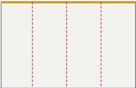
Ściana prawa od lewej: FR-003 ... FR-006, LED 390 × 250 cm plik 393 × 253 cm, spad 1,5 cm po obrysie, łączęń: 3
