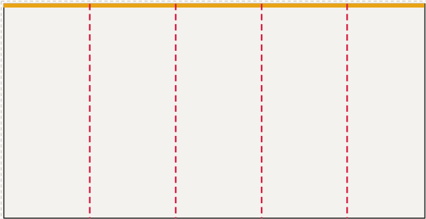
Ściana tylna od lewej: FR-001 ... FR-005, LED 490 × 250 cm plik 493 × 253 cm, spód 1,5 cm po obrysie, łączni: 4
