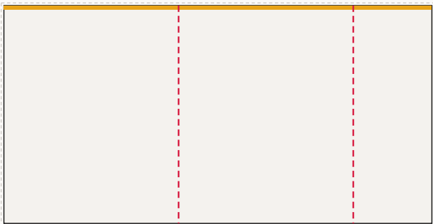
Ściana tylna od lewej: FR-001 ... FR-003, LED 490 × 250 cm plik 493 × 253 cm, spad 1,5 cm po obrysie, łączef: 2
