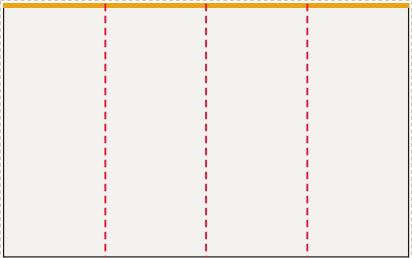
Ściana prawa od lewej: FR-005 ..., FR-008, LED 400 × 250 cm plik 403 × 253 cm, spad 1,5 cm po obrysie, łączeń: 3
