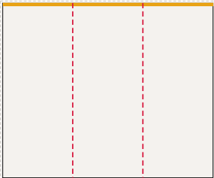
Regał Faro, strona A od lewej: IN-001 ... IN-003, LED 300 × 250 cm plik 303 × 253 cm, spad 1,5 cm po obrysie, łączęć: 2
