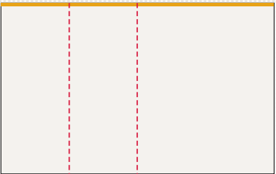
Ściana prawa od lewej: FR-007 ... FR-009, LED 400 × 250 cm plik 403 × 253 cm, spad 1,5 cm po obrysie, łącząc: 2
