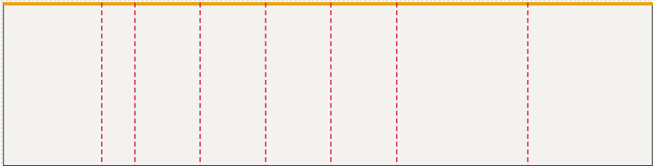
Ściana tylna od lewej: FR-001 ... FR-008, LED 990 × 250 cm plik 993 × 253 cm, spad 1,5 cm po obrysie, łączeń: 7
