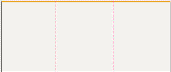
Ściana prawa od lewej: FR-009 ... FR-011, LED 590 × 250 cm plik 593 × 253 cm, spad 1,5 cm po obrysie, łączeń: 2
