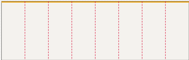
Ściana tylna od lewej: FR-001, ... FR-008, LED 800 × 250 cm plik 803 × 253 cm, spad 1,5 cm po obrysie, łączący: 7
