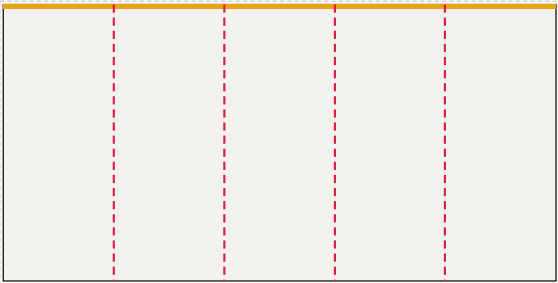
Ściana lewa od lewej: FR-010 ... FR-006, LED 500 × 250 cm plik 503 × 253 cm, spad 1,5 cm po obrysie, łączeń: 4
