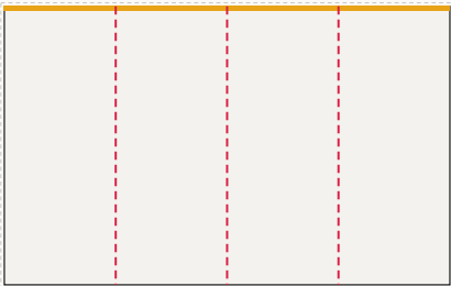
Ściana lewa od lewej: FR-008 ... FR-005, LED 400 × 250 cm plik 403 × 253 cm, spad 1,5 cm po obrysie, łącząc: 3
