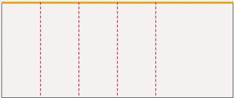
Ściana tylna od lewej: FR-002 ... FR-006, LED 600 × 250 cm plik 603 × 253 cm, spad 1,5 cm po obrysie, łączeń: 4
