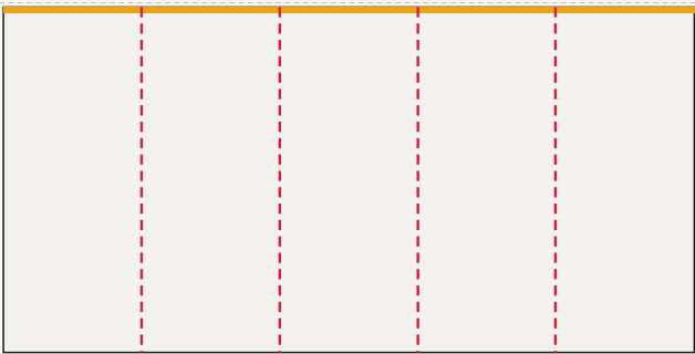
Ściana lewa od lewej: FR-007 ... FR-003, LED 500 × 250 cm plik 503 × 253 cm, spad 1,5 cm po obrysie, łączeń: 4
