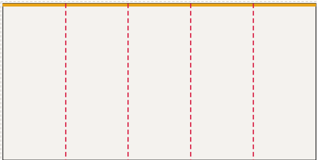
Ściana tylna od lewej: FR-002 ... FR-006, LED 500 × 250 cm plik 503 × 253 cm, spad 1,5 cm po obrysie, łączeń: 4
