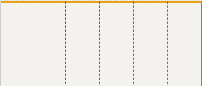
Ściana tylna od lewej: FR-001 ... FR-005, LED 590 × 250 cm plik 593 × 253 cm, spąd 1,5 cm po obrysie, łączeń: 4
