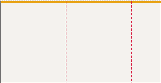
Ściana lewa od lewej: FR-008 ... FR-006, LED 490 × 250 cm plik 493 × 253 cm, spąd 1,5 cm po obrysie, łączeń: 2
