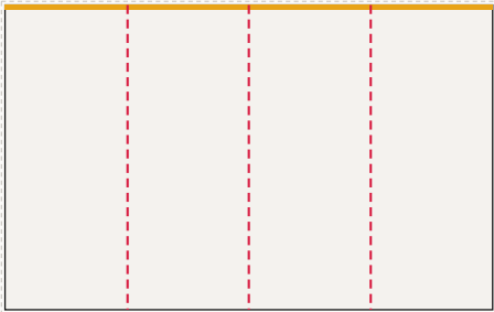
Ściana tylna od lewej: FR-002 ... FR-005, LED 400 × 250 cm plik 403 × 253 cm, spąd 1,5 cm po obrysie, łączeń: 3
