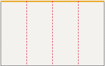
Ściana lewa od lewej: FR-009 ... FR-006, LED 400 × 250 cm plik 403 × 253 cm, spad 1,5 cm po obrysie, łączeń: 3
