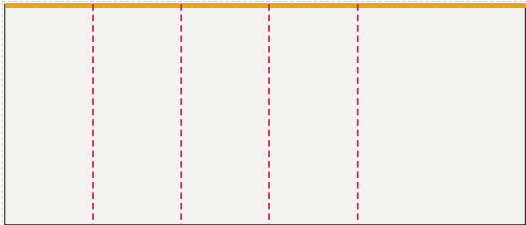
Ściana lewa od lewej: FR-010 ... FR-006, LED 590 × 250 cm plik 593 × 253 cm, spad 1,5 cm po obrysie, łączący: 4
