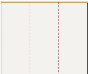
Regal Faro, strona A od lewej: IN-001 ... IN-003, LED 300 × 250 cm plik 303 × 253 cm, spad 1,5 cm po obrysie, łączeń: 2
