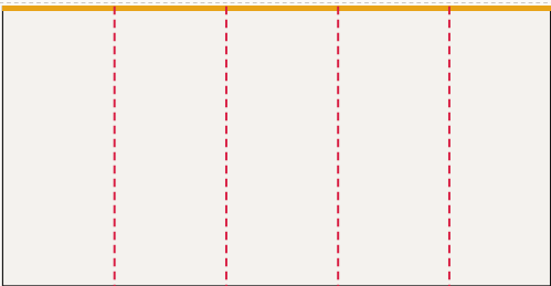
Ściana lewa od lewej: FR-009 ... FR-005, LED 490 × 250 cm plik 493 × 253 cm, spad 1,5 cm po obrysie, łączęć: 4
