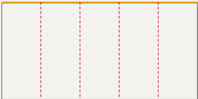
Ściana tylna, część 1 z 2 od lewej: FR-001 ... FR-005, LED 500 × 250 cm plik 503 × 253 cm, spad 1,5 cm po obrysie, łączeń: 4
