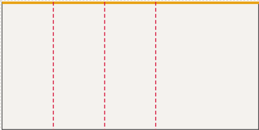
Ściana lewa od lewej: FR-006 ..., FR-003, LED 500 × 250 cm plik 503 × 253 cm, spad 1,5 cm po obrysie, łączeń: 3
