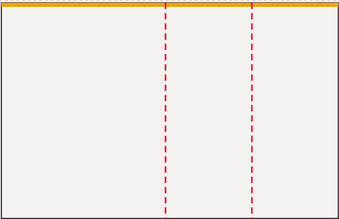
Ściana prawa od lewej: FR-007 ... FR-009, LED 390 × 250 cm plik 393 × 253 cm, spad 1,5 cm po obrysie, łączeń: 2
