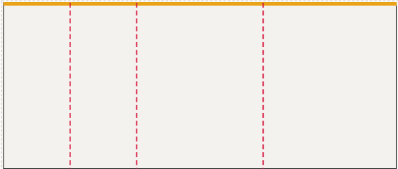
Ściana lewa od lewej: FR-010 ... FR-007, LED 590 × 250 cm plik 593 × 253 cm, spad 1,5 cm po obrysie, łączę: 3
