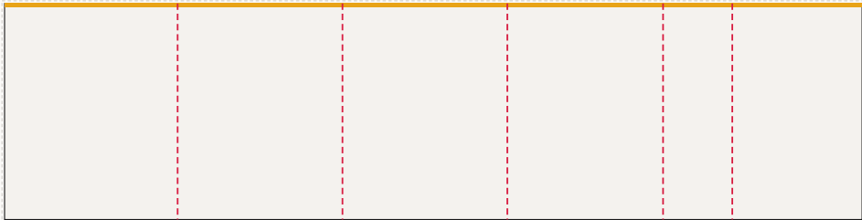
Ściana tylna od lewej: FR-001 ... FR-006, LED 991 × 250 cm plik 994 × 253 cm, spad 1,5 cm po obrysie, łączę: 5
