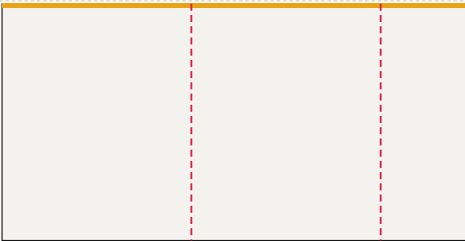
Ściana lewa od lewej: FR-011 ... FR-009, LED 490 × 250 cm plik 493 × 253 cm, spad 1,5 cm po obrysie, łączęć: 2
