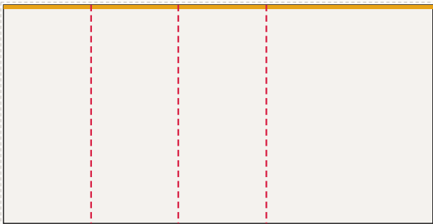
Ściana lewa od lewej: FR-009 ... FR-006, LED 490 × 250 cm plik 493 × 253 cm, spad 1,5 cm po obrysie, łączni: 3
