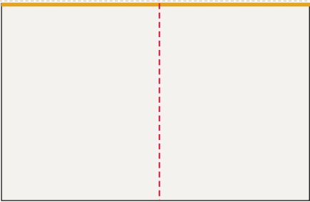
Ściana lewa od lewej: FR-005, FR-004, LED 390 × 250 cm plik 393 × 253 cm, spąd 1,5 cm po obrysie, łączeń: 1
